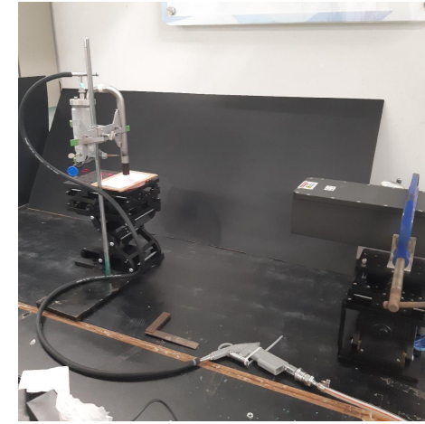
2D Mini Laser Doppler Velocimetry
